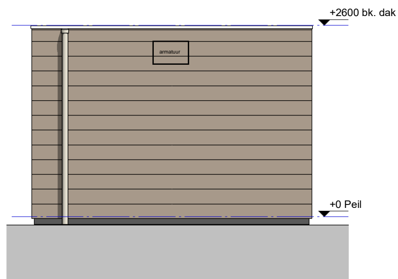
achtergevel
