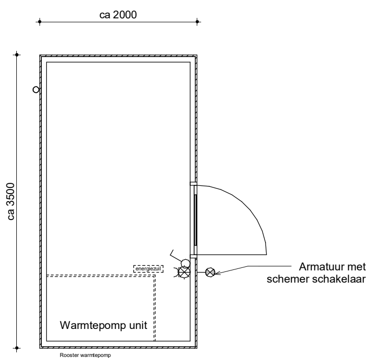
Begane grond
