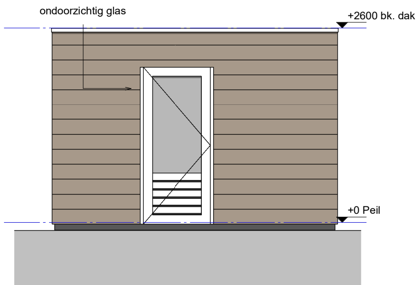
voorgevel
