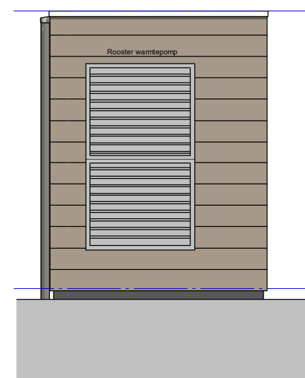
linkergevel
