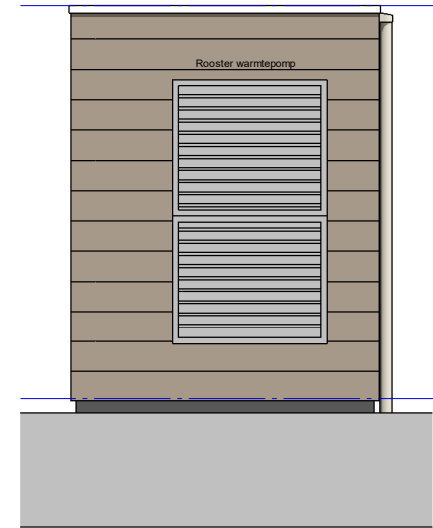
rechtergevel
